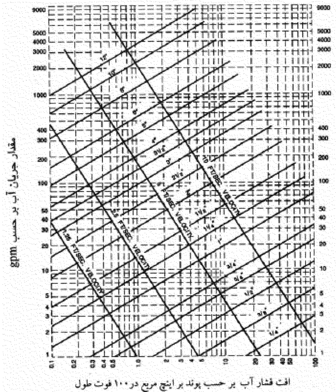
شکل پ ۵-۵-۱ (IP) منحنی اندازه گذاری لوله‌های مسی نوع K از استاندارد ANSI B 88
