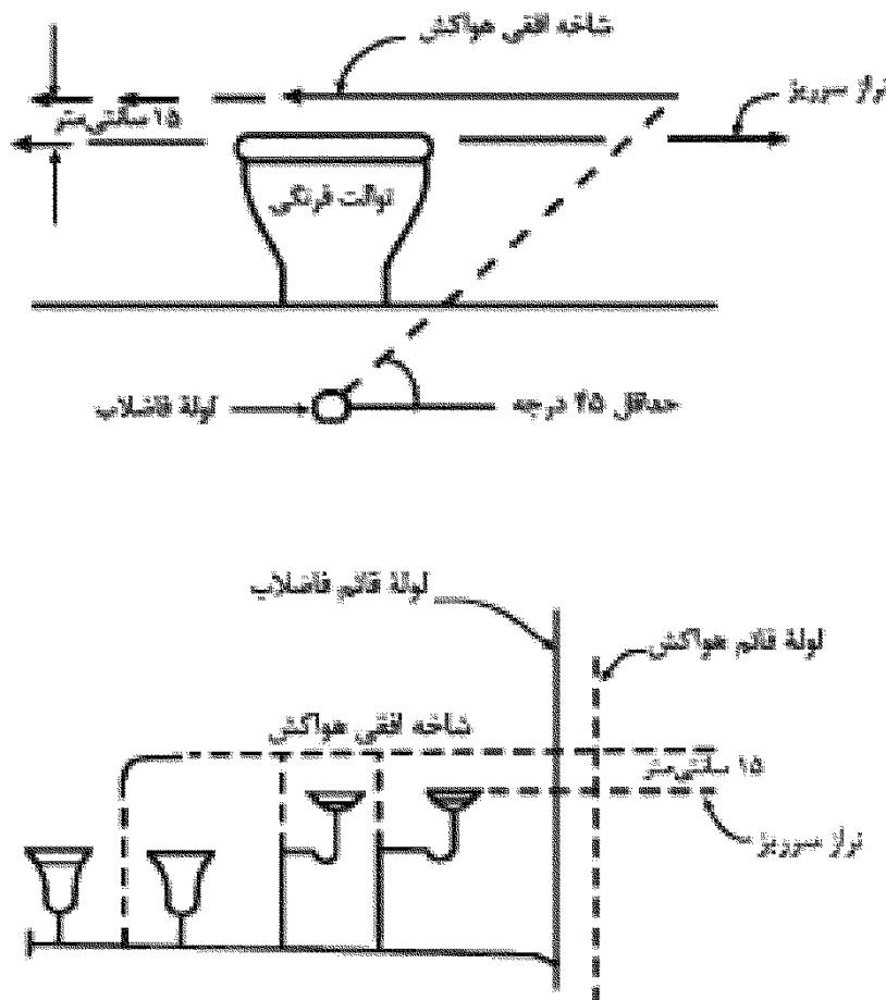
شکل شماره (۱۶-۶-۲-۵) "پ" (۲): اتصال هواکش به شاخه افقی لوله فاضلاب
